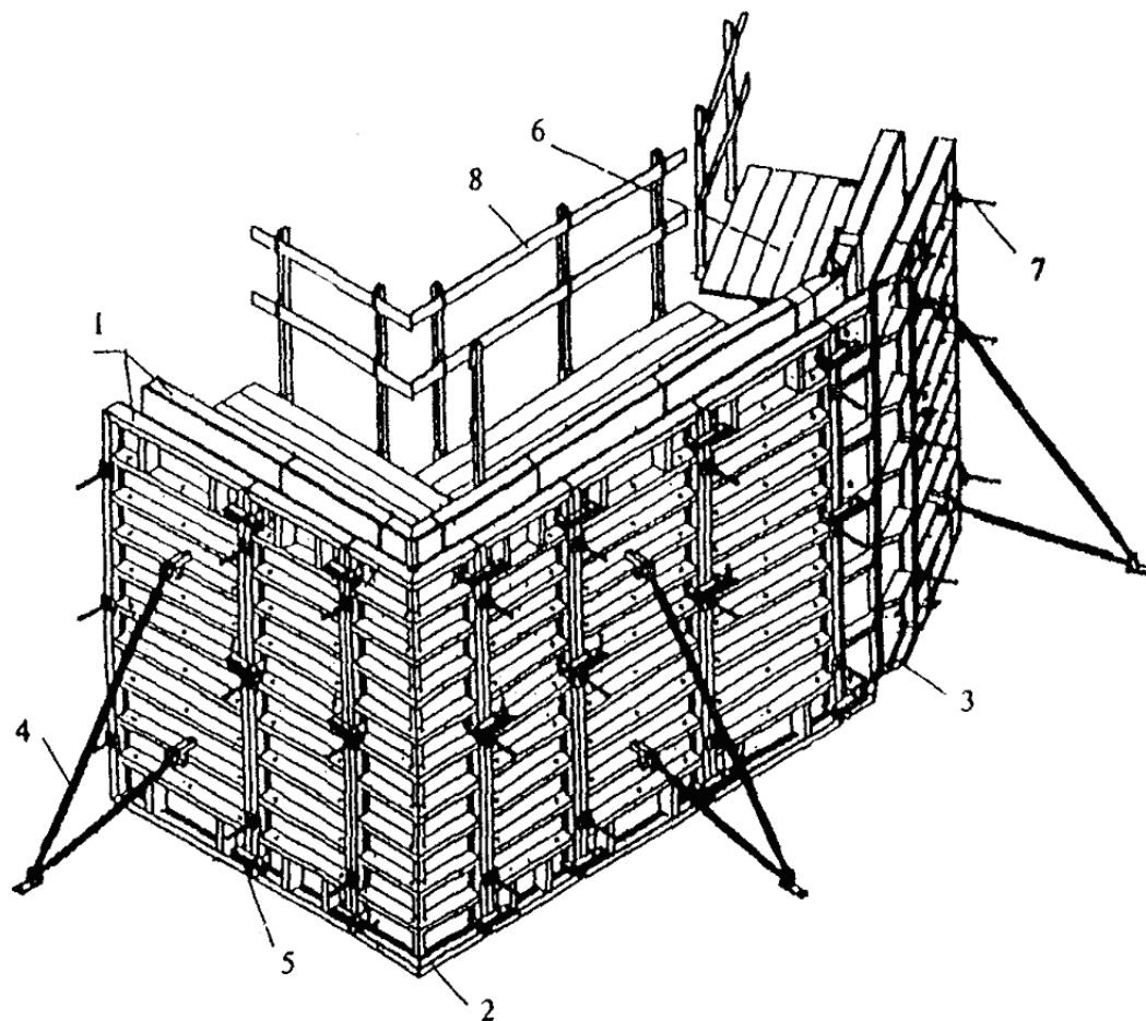
Рисунок А.4 - Мелкощитовая разборная опалубка перекрытий (на стойках)
