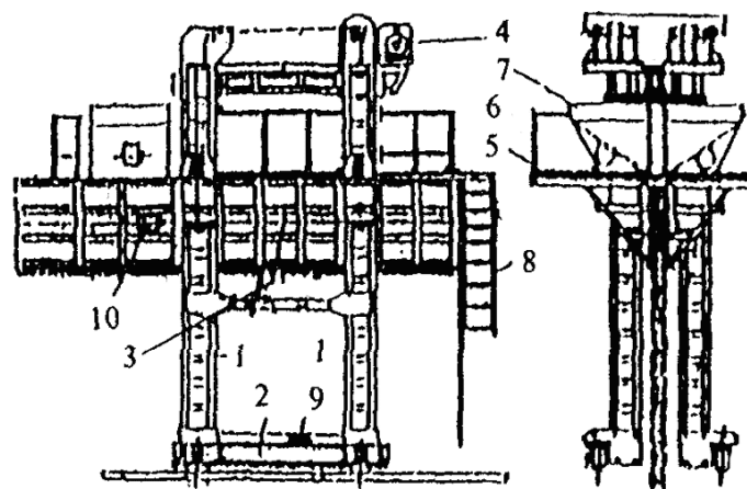
Рисунок А.13 - Скользящая опалубка
