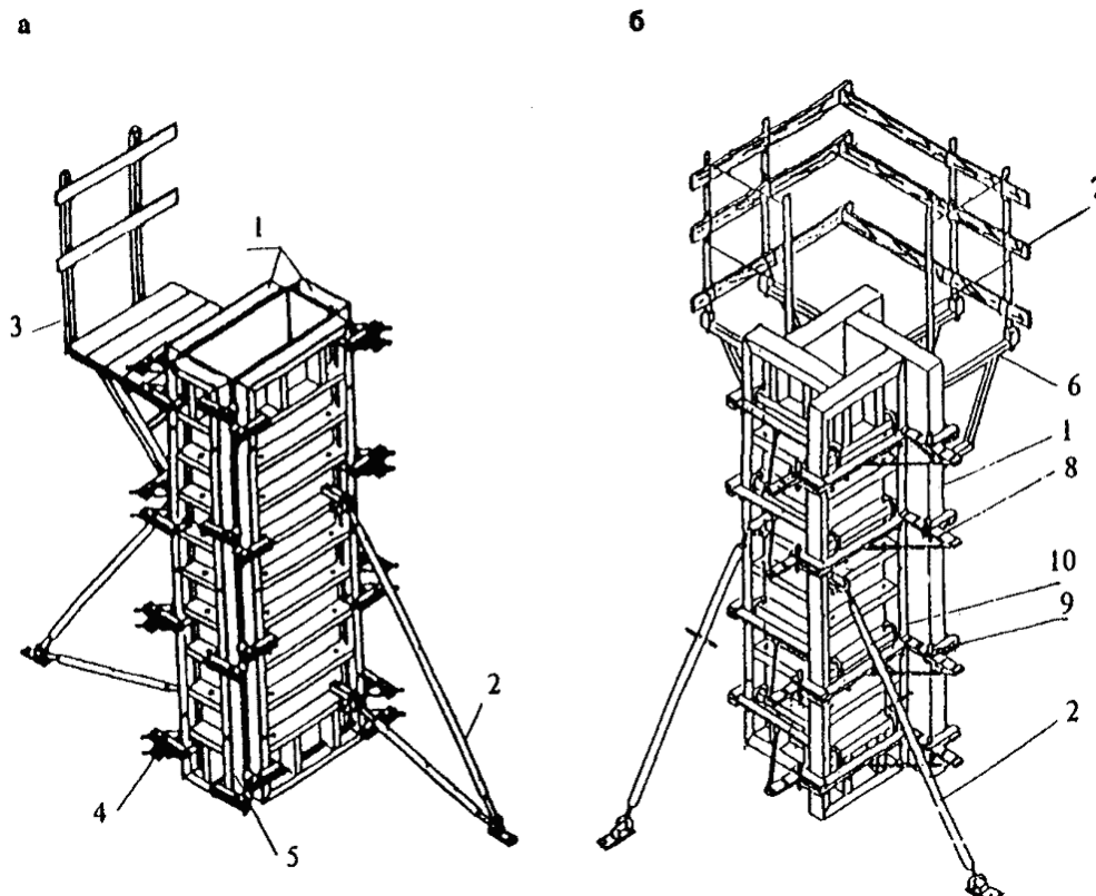
Рисунок А.6 - Крупнощитовая модульная опалубка стен (с наружными подмостями для бетонирования наружной, фасадной, торцевой стен)
