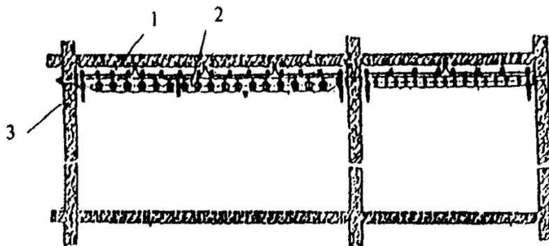
Рисунок А.8 - Крупнощитовая разборная опалубка стен
