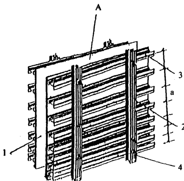
Рисунок А.7 - Крупнощитовая модульная опалубка колонн
